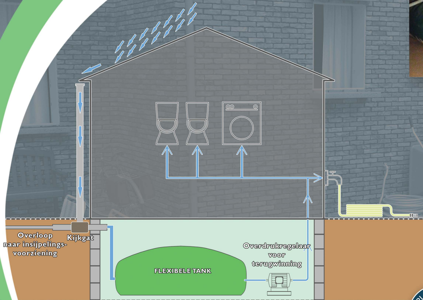
Hydraulisch schema voor hergebruik van regenwater
